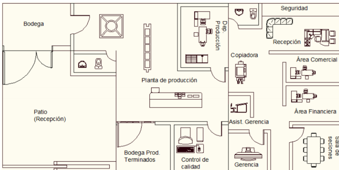
Ilustración 9. Distribución de Planta
